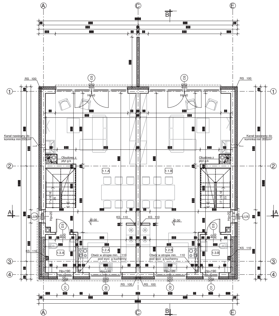
ZESTAWIENIE POMIESZCZE - PARTER - SEGMENT A
