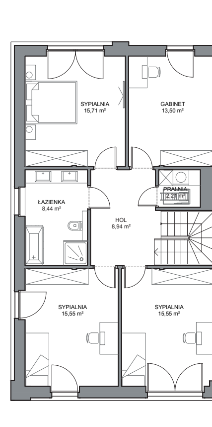
PIĘTRO 79,60 m 2
