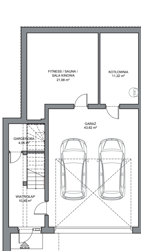
PIWNICA 91,37 m 2
